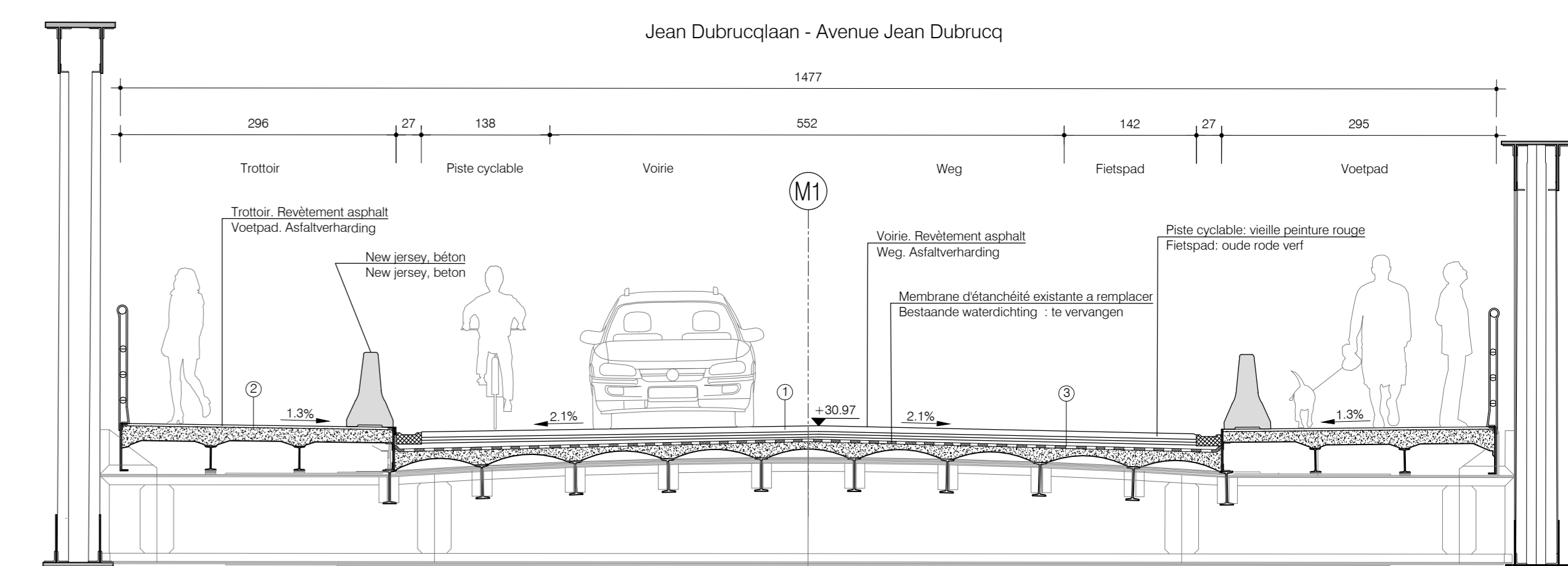
Section A-A: Coupe transversale / Dwarssnede Ech/Sch. 1:50
