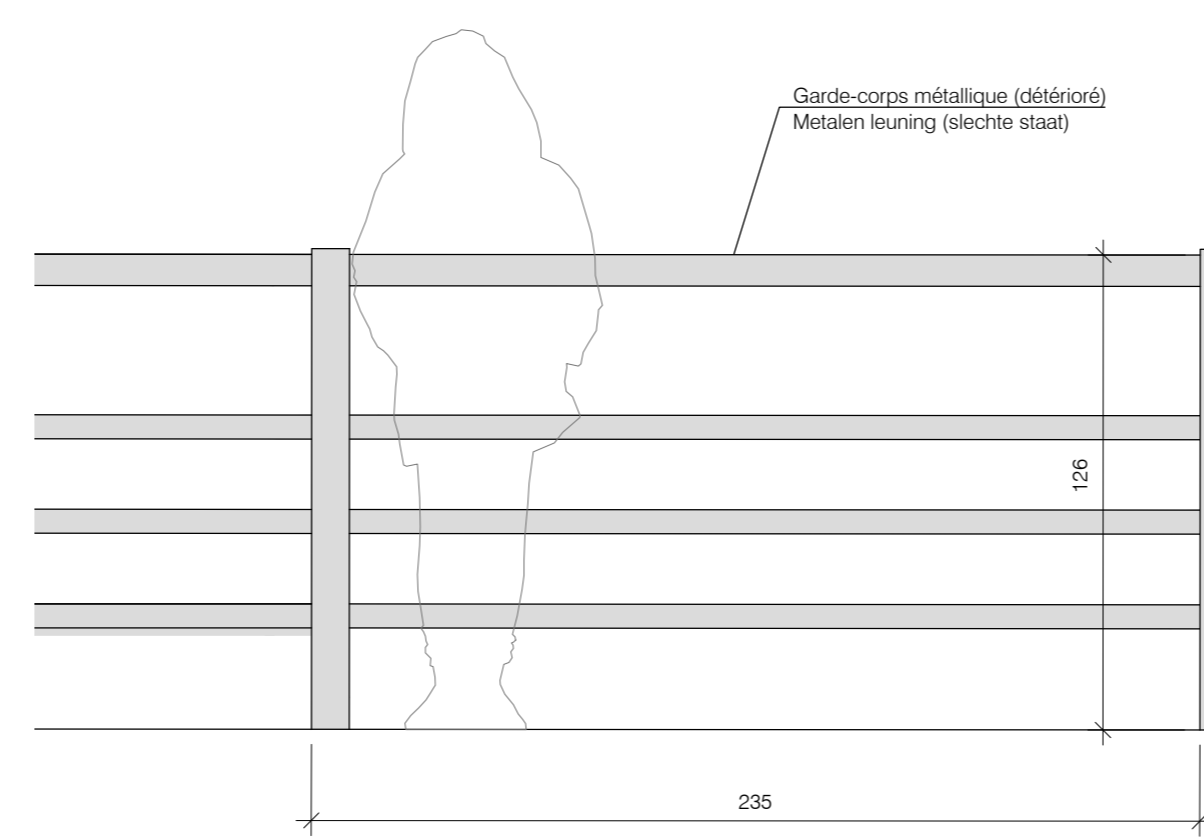
Detail: Garde-corps existant / Bestaande leuning Ech / Sch. 1:20
